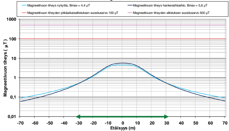
Magneettikenttä
