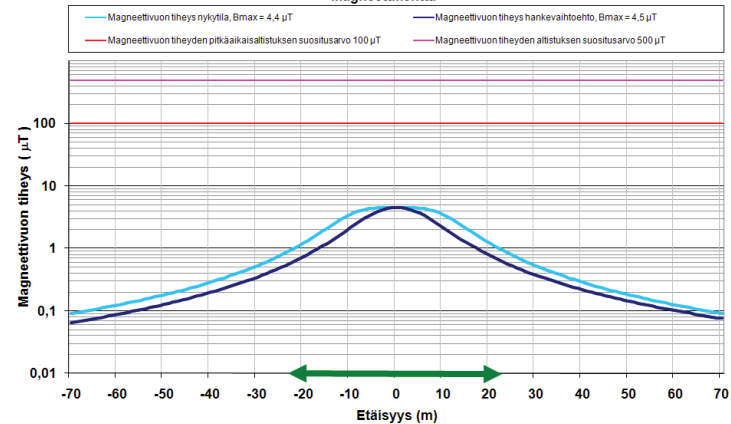
Magneettikenttä
