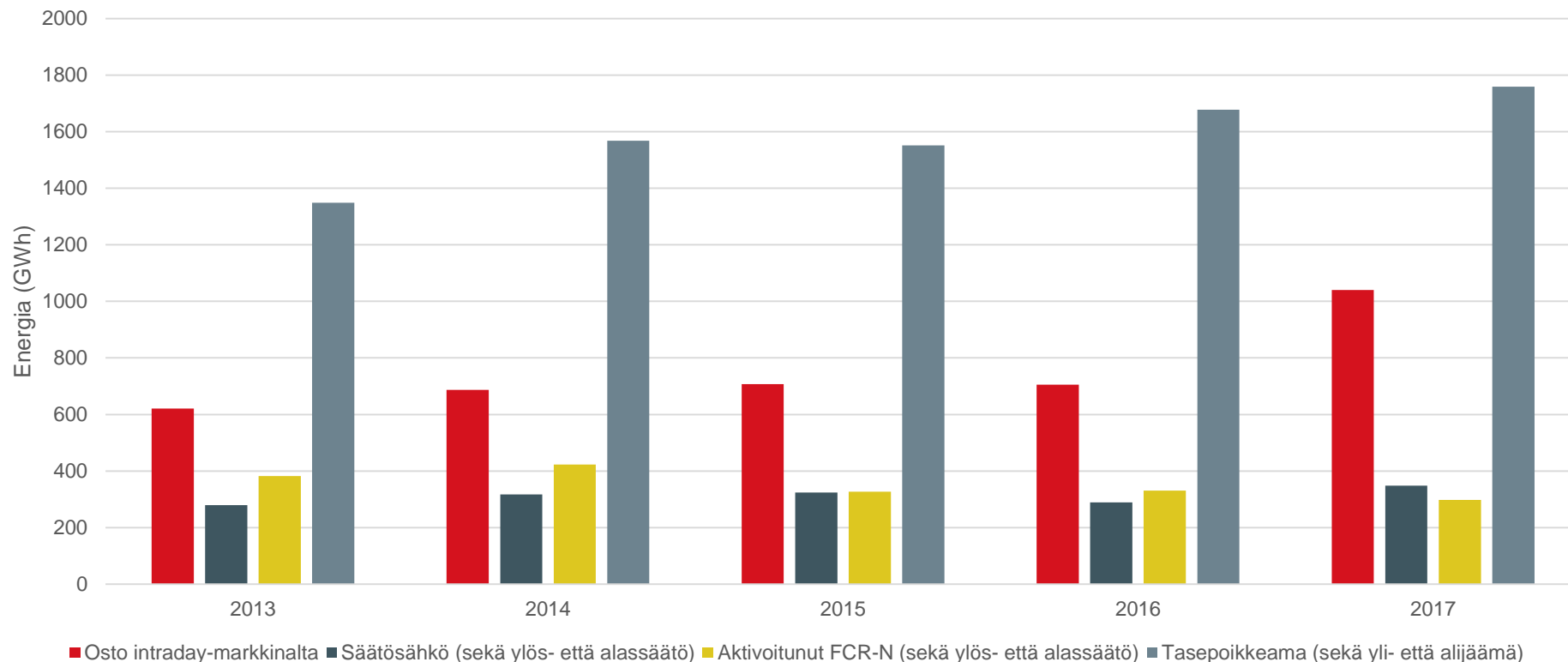
Vuosittainen sähköenergian määrä Suomessa
