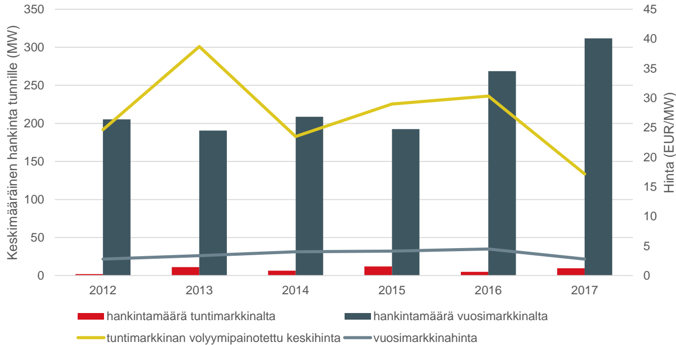
Toteutunut vuotuinen FCR-D hankinta
