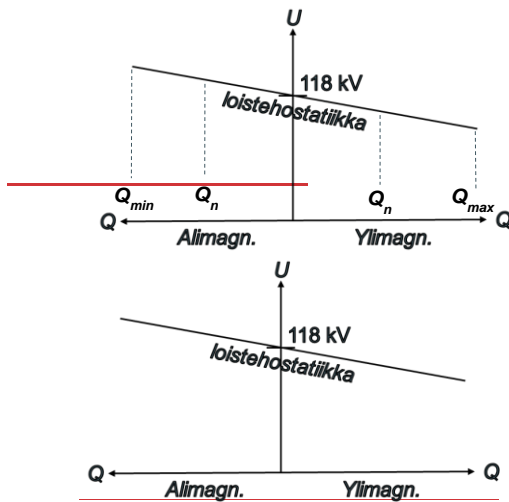
Kuva 21.1. Loistehostatiikka
