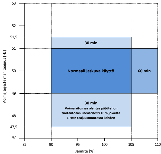
Kuva 10.57. Voimalaitoksen on pysyttävä verkkoon kytkeytyneenä kuvassa esitetyillä erilaisilla liittymispisteiden taajuuksilla ja jännitteillä. Jatkuvan toiminta-alueen 100 %:n jännite on 400 kV:n verkossa aina 400 kV. Muilla jännitteillä 100 %:n arvoa vastaava jännite on selvitettävä liittymispisteiden verkonhaltijalta.
