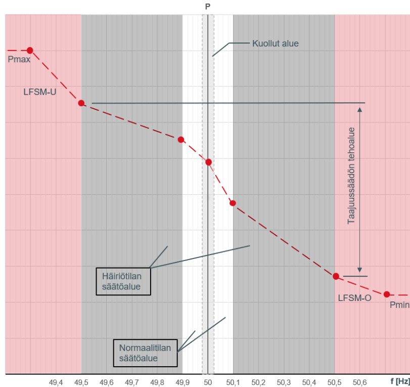
Kuva 16.1. Tajuuksäädön jatkuva toiminta eri taajuusalueilla. Kaikille taajuusalueille on omat statiikka- ja tehoraaja-asettelunsa. Kuollut alue 50 Hz:n ympärillä on aseteltavissa erikseen. Kuvassa esitetyt taajuusarvot, statiikka-asettelut ja tehoalueet ovat esimerkinomaisia. Tehotasot P_{max} ja P_{min} kuvaavat suurinta ja pienintä säätötasoa.
