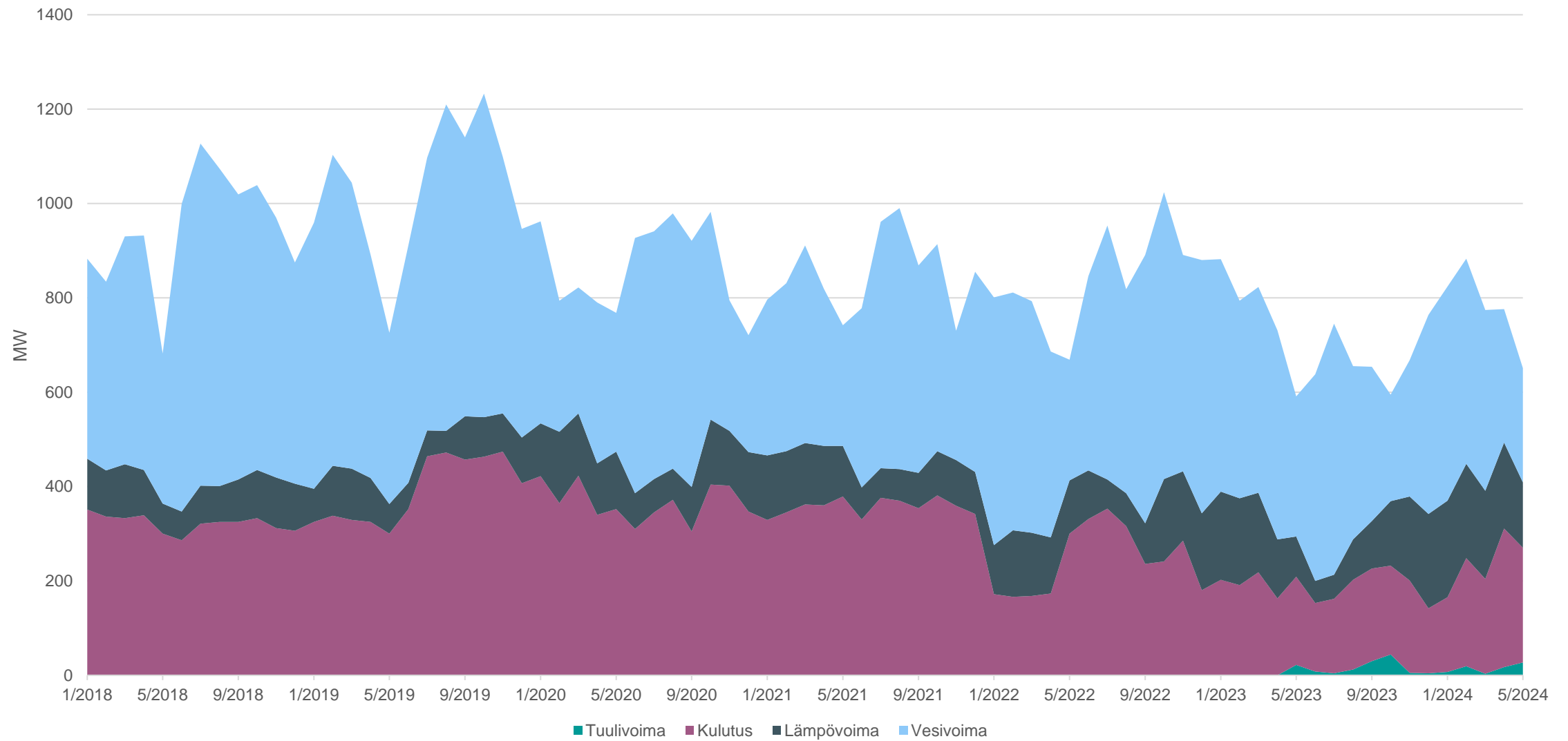
mFRR ylös kuukausittainen tarjousmäärä teknologioittain ka. (MW), 1/2018-5/2024
