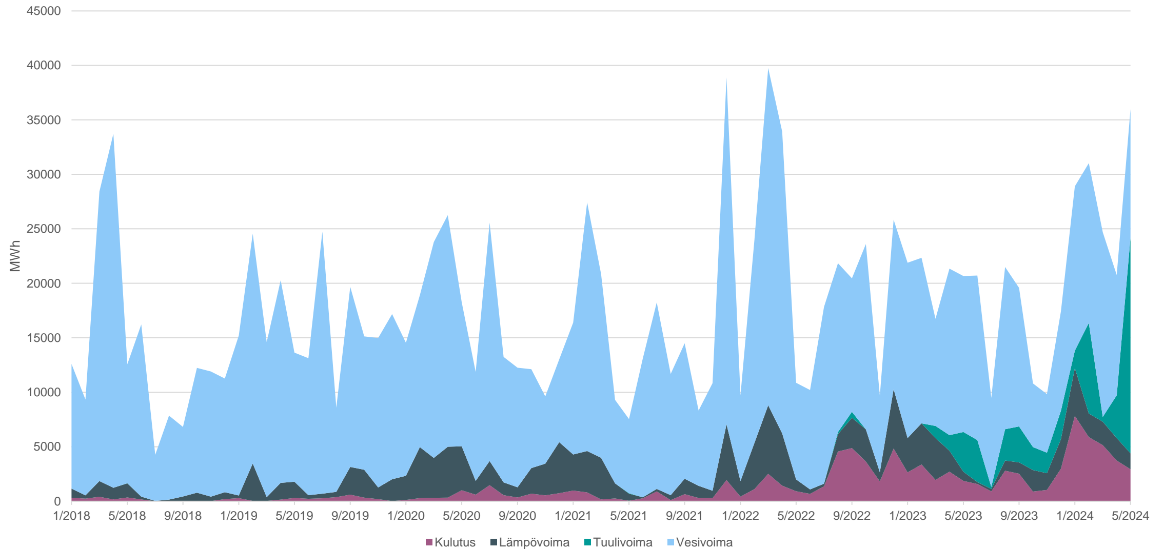
mFRR alas kuukausittainen aktivoitu energiasumma teknologioittain (MWh), 1/2018-5/2024
