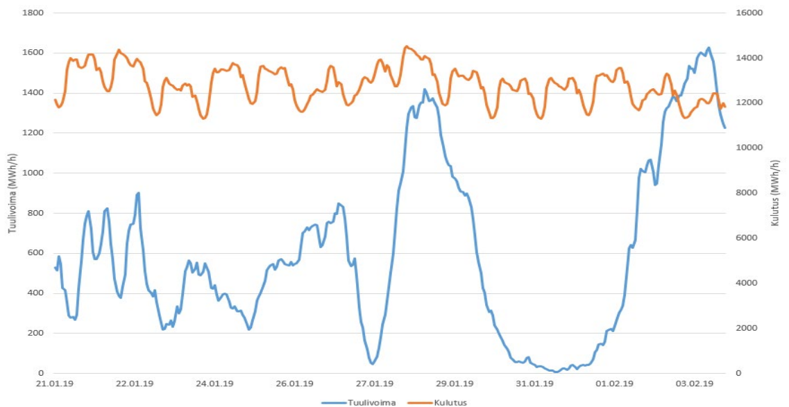
Kuva 7. Tuulivoiman tuotanto ja sähkön kulutus Suomessa viikoilla 4-5/2019.
